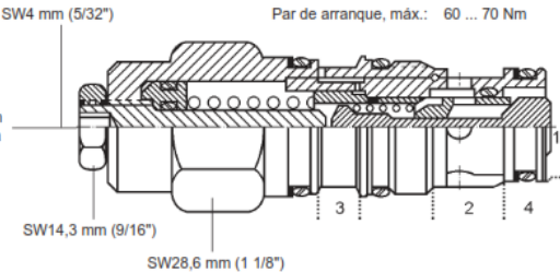
Válvula de freno de bajada CBDD LJN
