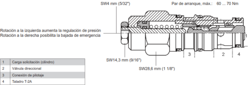
Válvula de freno de bajada CBDD LNJ
