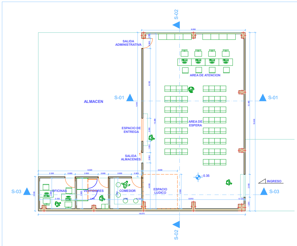
0. VISTA EN PLANTA 1:100
