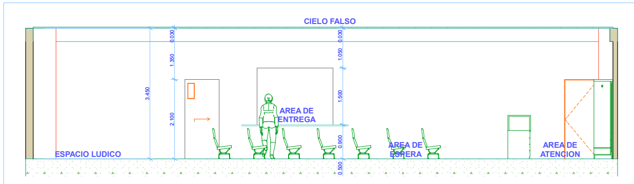
S-02 CORTE LONGITUDINAL 1:50
